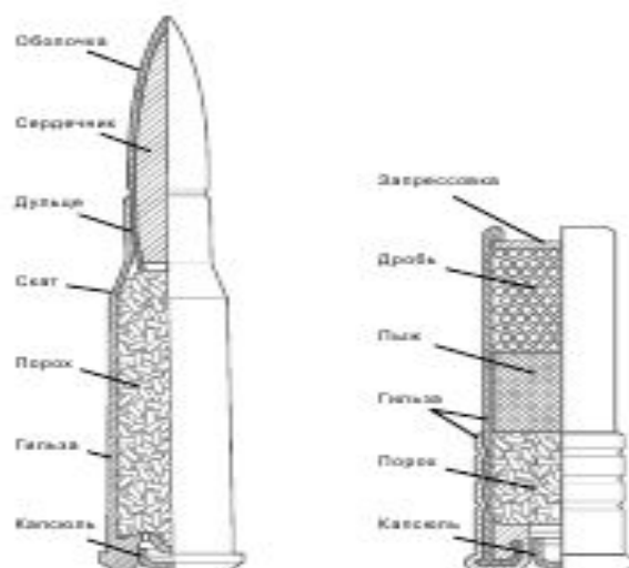
Схема патронов для гладкоствольного (справа) и нарезного оружия
